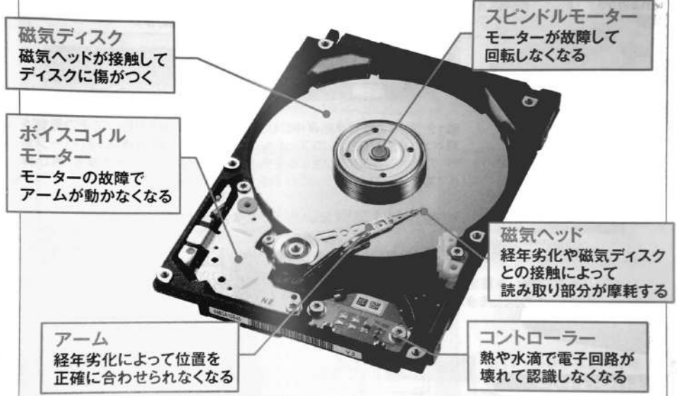
図1 HDD (ハードディスクドライブ)は磁気ディスクやアーム、各種モーターなどの機械駆動部品を多く含む精密機械であるため、モーターなどの不具合のほか、磁気ディスクについたわずかな傷などが故障につながる。なぜHDDが壊れやすいのかを詳しく見ていこう
